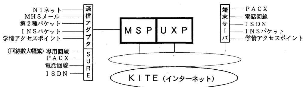
次期システムのネットワーク構成
